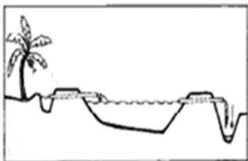
Figure 16: Etang partiellement creusé et endigué (Source : Doc Dac_MEN)
