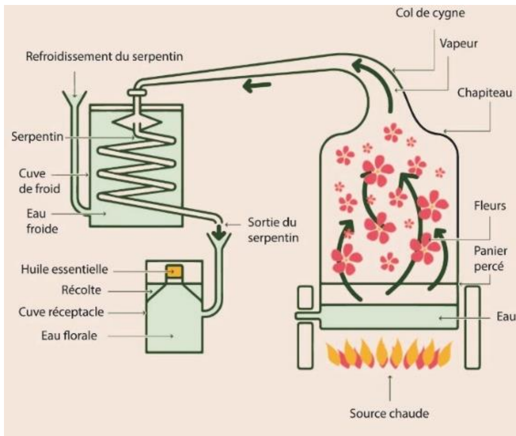
Figure 2: Distillation d'hydrolat avec un alambic
