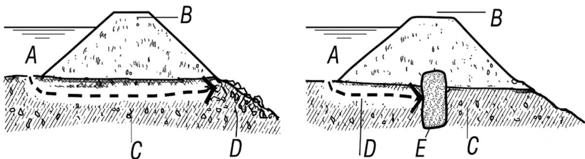
Figure 18: Le noyau en argile (Source : Doc Dac_MEN)
