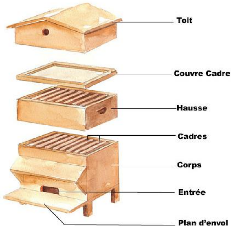
Figure 24: Les composants d'une ruche à cadre
