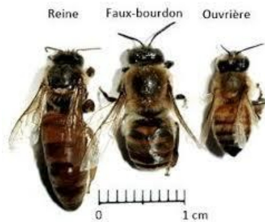
Figure 20 : Les trois types d'abeille
