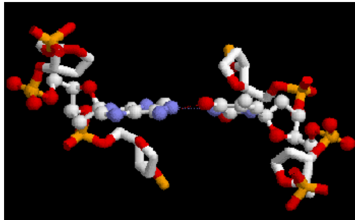
Paire de bases AT, vue de profil
