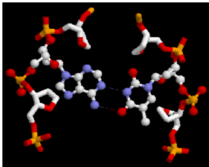
Paire de bases AT, vue de dessus
