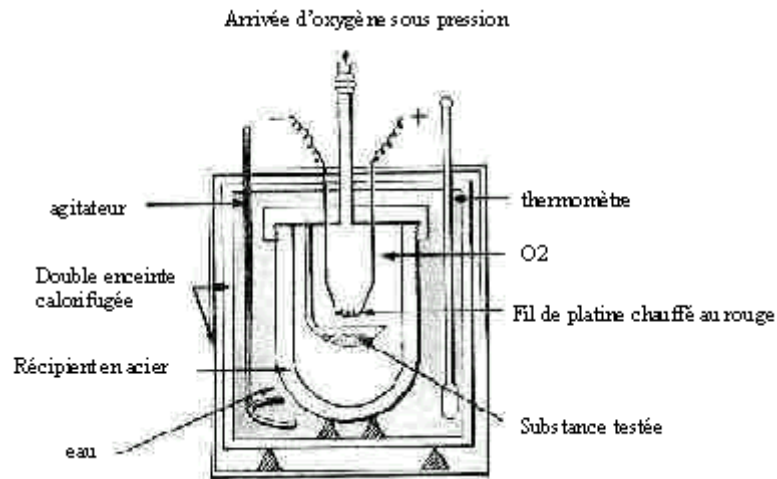
Document 1 : Bombe calorimétrique dans son calorimètre
