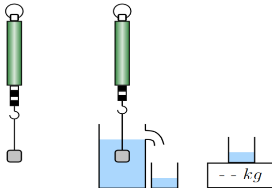
Mesure du poids de liquide d plac 
