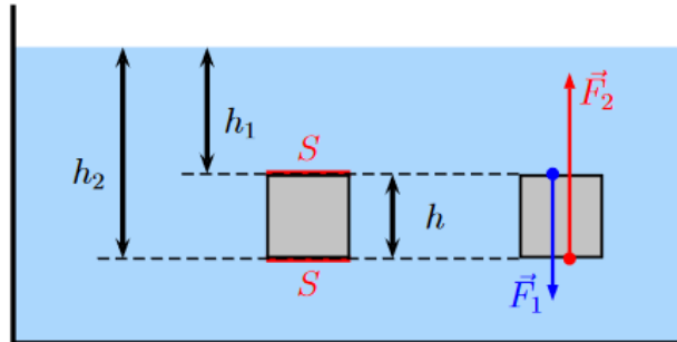
Un parallélépipède immergé dans un liquide
