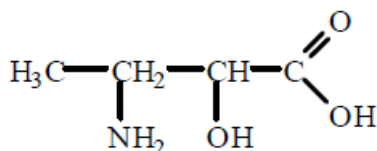
Acide 3-amino-2-hydroxybutanoïque
