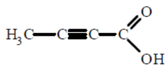
Acide but-2-ynoïque
