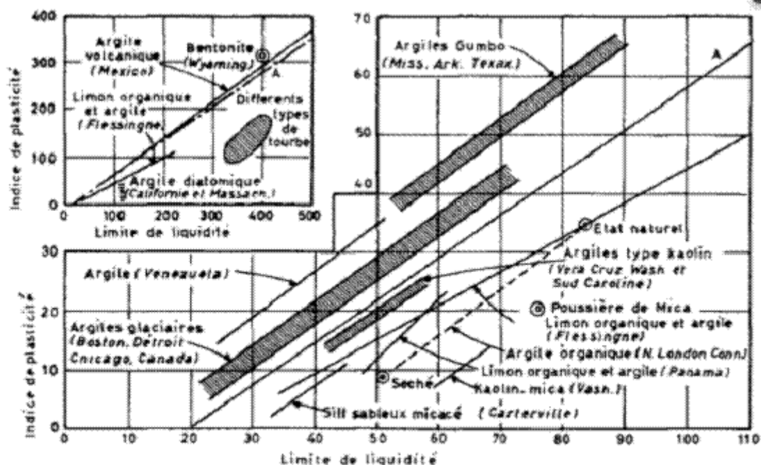
Fig. 1a - Relation entre la limite de liquidité et l'indice de plasticité pour des sols caractéristiques.
