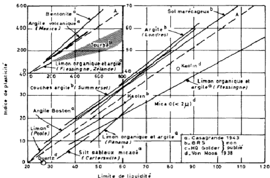
Fig. 1b - Relation entre la limite de liquidité et l'indice de plasticité.
